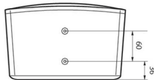
底面
